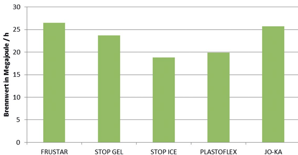
Brennwert einer Frostschutzkerze pro Stunde in MJ
